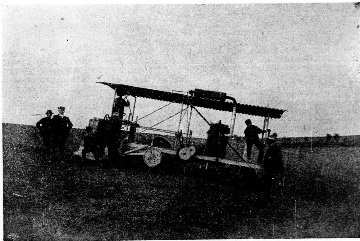
A Kőszegi-féle motoros talajművelő gép lejtőn letelé állva. A gép elején látható a hárcmhengeres benzínmotor.
