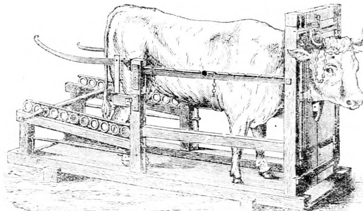
Kalodaszerkezet ökörpatkoláshoz.
