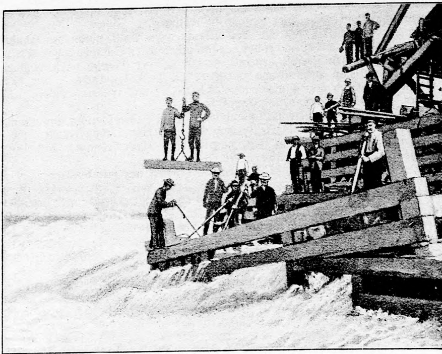
Die neuen Arbeiten am Niagara: Ein gefährlicher Arbeitsplan. (Mit Text.) Nicht über den niederfallenden Wasserfällen.
