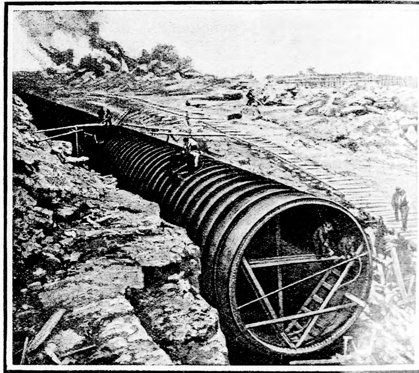
Die neuen Arbeiten am Niagara: Hauptrohrleitung von 6 Meter Durchmesser zur Fortführung der Wasserfälle. (Mit Text.)
