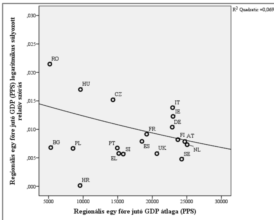
4. ábra: Williamson-görbe, 2000
