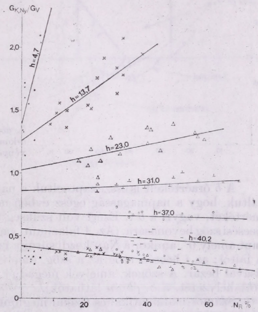
5. ábra: G_{KNy}/G_V változása a relatív napfénytartam függvényében, különböző napmagasságoknál, ha G_V = Direkt + Diffúz, és napmagasságtól függetlenül, ha G = Diffúz
