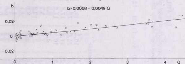
9. ábra: \Delta G_{KN_y}/G_A = a + b N_R összefüggés irányteng- sének függése a Nap és fal re- latív helyzetét meghatározó Q paramétértől; a korrelációs együttható, r = 0.866
