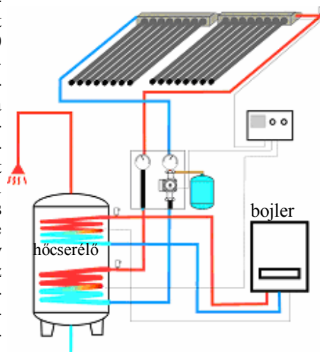
Napkollektor melegvíz készítésre bekötve
