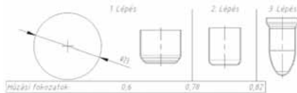
5.kép Első technológiai sorrend
