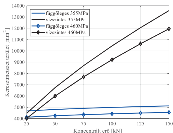
10. ábra Optimális keresztmetszet területek koncentrált terhelés és szélterhelés esetén
