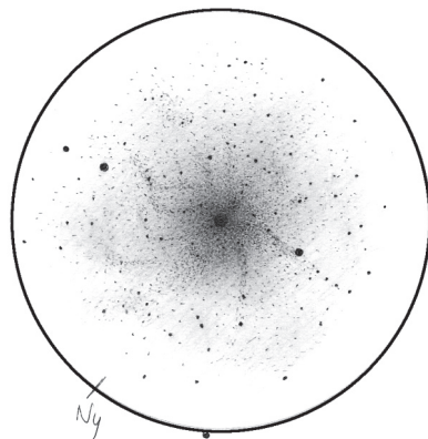
Az égbolt második legfényesebb gömbhalmaz, a 47 Tucanae Sánta Gábor rajzán (13 T, 108x, 31')
