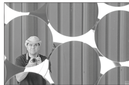
A kisebb méretű HESS távcsövek tükrei kerek formájúak, és 50 cm-es átmérőjűek: egyetlenegynek nagyobb a felülete, mint az expedícióra elvitt összes optikai eszközünké együttvéve
