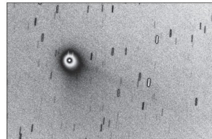
Kuli Zoltán május 19-én hajnalban készült 38,5 perces felvételének ekvizitogramján jól látható a Lemmon-üstökös ion- és porcsóvája is (102/500 L, Nikon D5100, ISO 3200)
