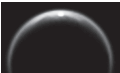
A Cassini-szonda felvétele egy Titan felszínén levő tó tükörn megcsillanó napfényről
