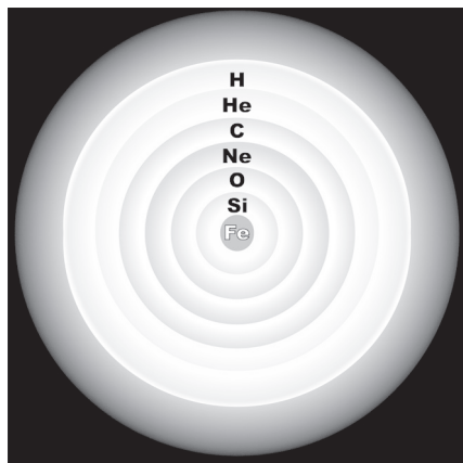
A nagy tömegű csillagok fősorozat utáni fejlődésének végére kialakuló, hagymahéj-szerkezet (en.wikipedia.org)
