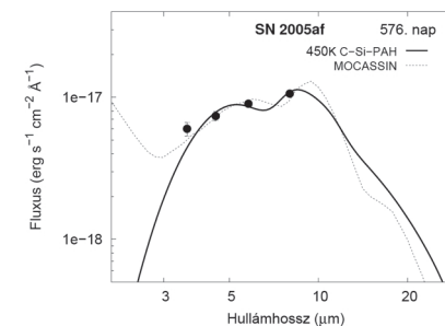
Az SN 2005af jelű szupernóva közép-infravörös spektrális energieleoszlása (fekete pöttyök), valamint az erre legjobban illeszkedő analitikus (folytonos vonal) és numerikus (szaggatott vonal) pormodell, szilikáttartalmú porösszetétel esetén
