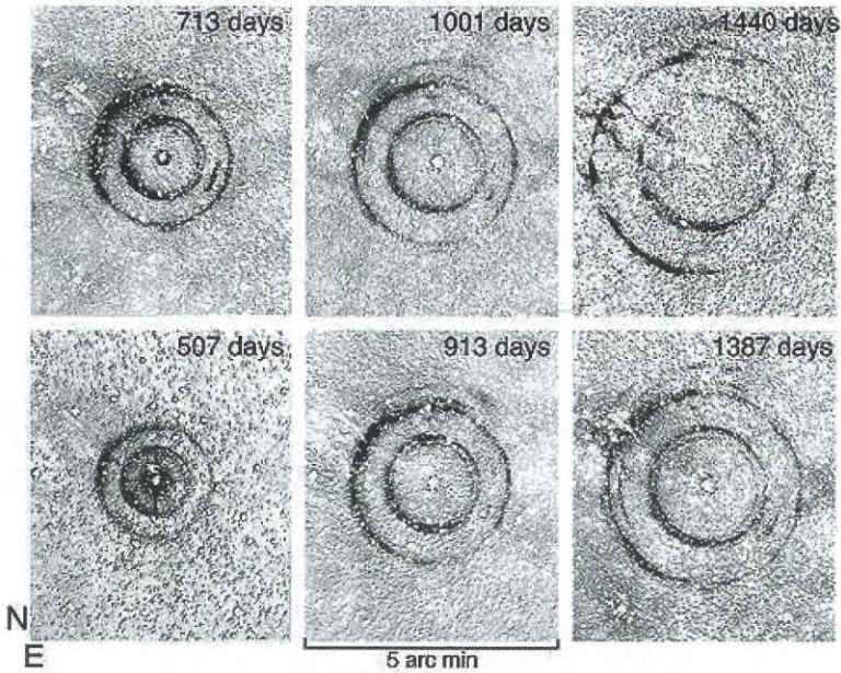
Az SN 1987A visszfénye az Angol-Ausztrál Teleszkóppal készített fotókon. Az igen halvány gyűrűk kimutatásához a fél órás expozíciós idejű fényképeket digitalizálták, majd kivonták belőlük a korábbi referenciaképet. Egy kép 5 ívperc széles, a számok a maximumtól eltelt napokat mutatják
