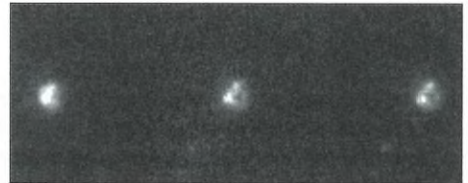
Az SN 1991T visszfényének változásai 1996 és 1998 között. A jobb oldali képen mérete 0,4''
