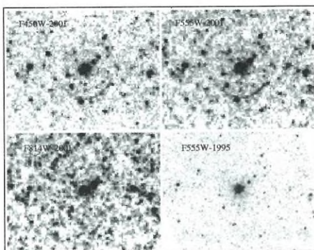
Az SN 1993J visszfényének ívdarabjai. A képek 10'' \times 10'' égtérületet mutatnak
