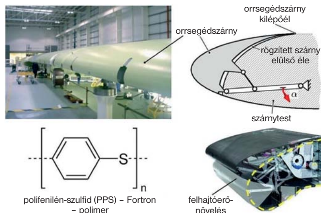
11. ábra. A szárny belépőélének (orrségédszárny) kialakítása, működése
