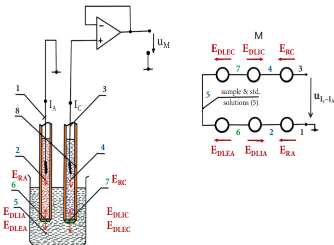
1. ábra. A szembekapcsolt anion- és kationszelektív elektródos mérőcella egyszerűsített működési vázlata és statikus elektromos helyettesítő képe
