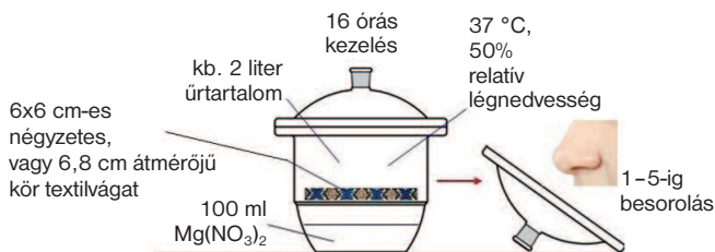
6. ábra. Szagvizsgálat az SNV 195651 szabvány szerint
