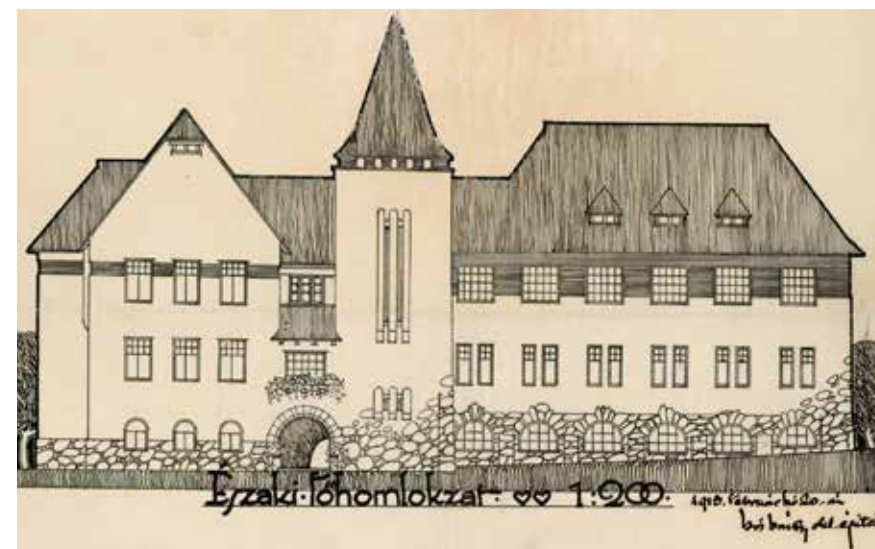
▼ Anya- és csecsemővédelmi pavilon terve, Vármegyei Közkórház, Sepsiszentgyörgy. Északi homlokzat terve, 1918. MÉM MDK
