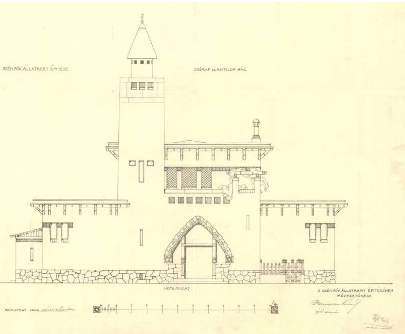
▲ Az állatkerti Zsiráfház terve, homlokzat, 1909. Budapest Főváros Levéltára
