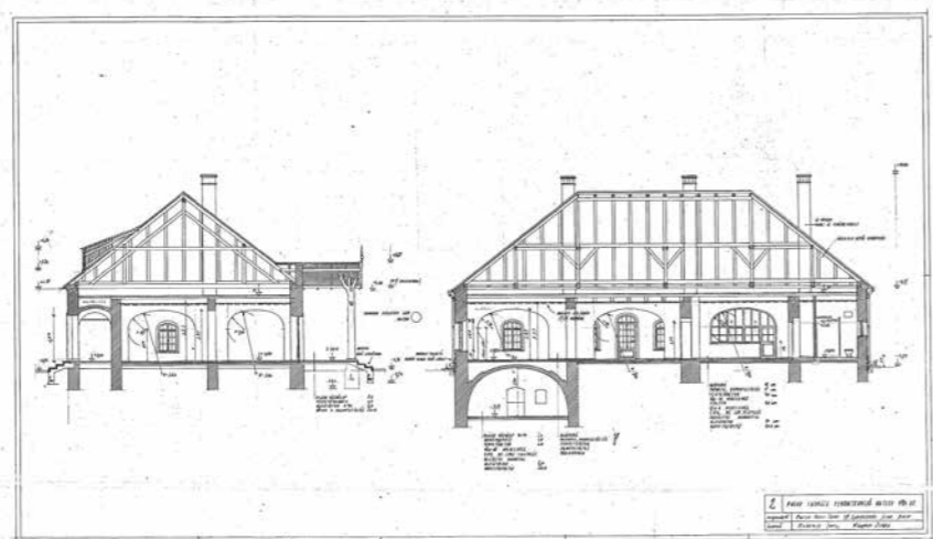
▲ Metszetek, Bagod
