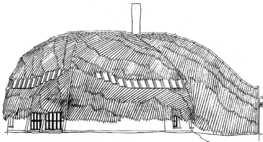
Homlokzati terve és homlokzati részletképzés. Faluház, Bak. Fotó: Gál Roland
