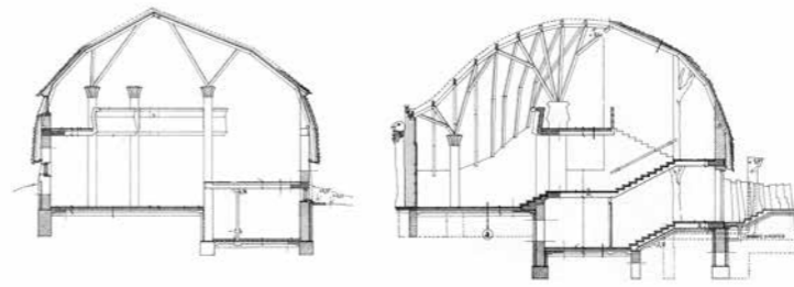
▲ Metszetek, faluház, Bak
