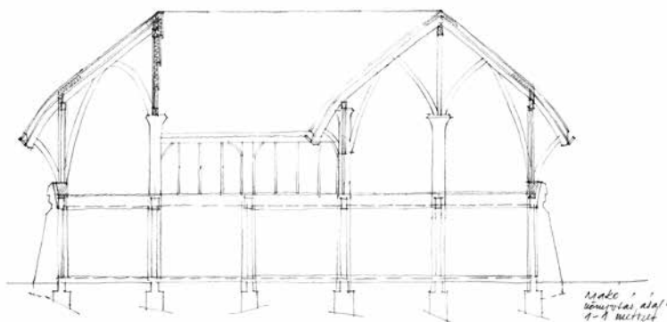
▲ Metszet. Makovecz Imre vázlata
