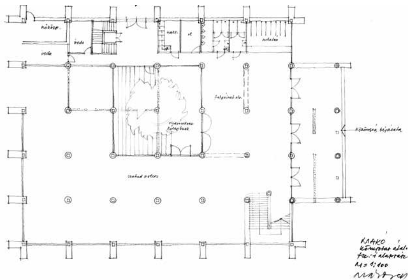
▲ Földszinti alaprajz. Makovecz Imre vázlata
