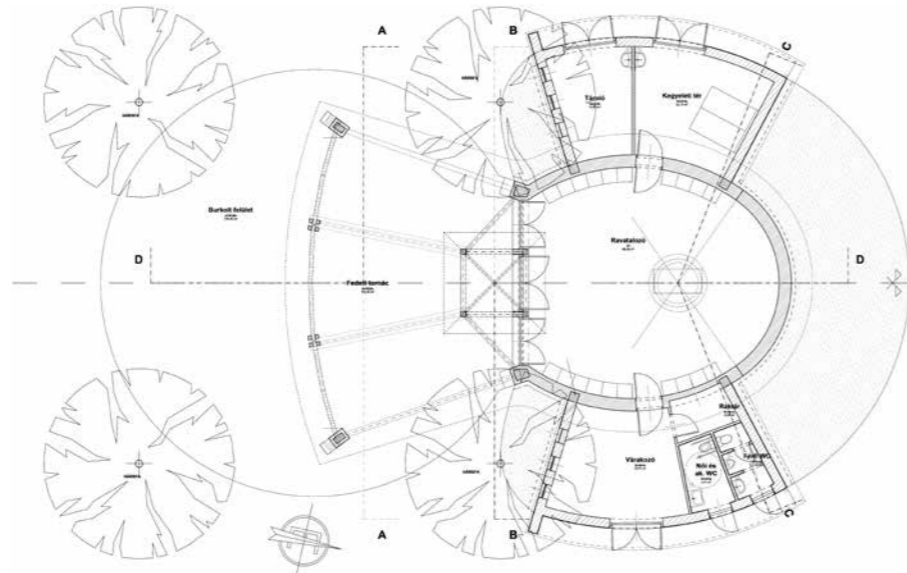
▲ Alaprajz
