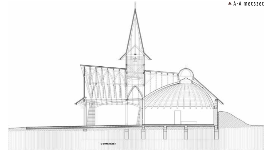
▲ D-D metszet
