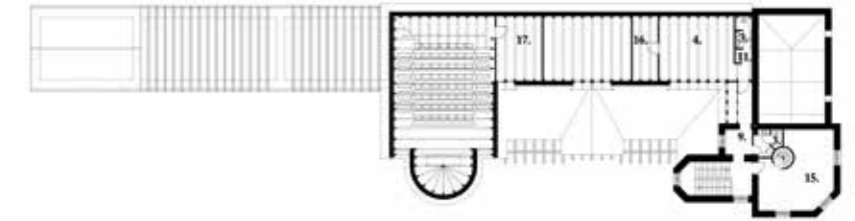
▲ Emeleti alaprajz
