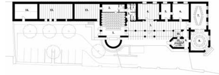
▲ Földszinti alaprajz
