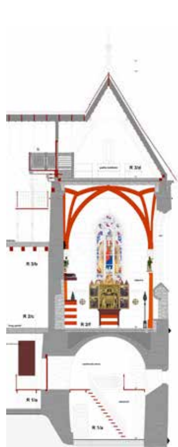
▲ Kápolna, keleti falnézet
