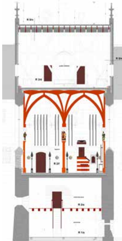
▲ Kápolna, északi falnézet
