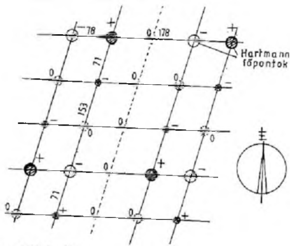
Hartmann-háló alaprajza
