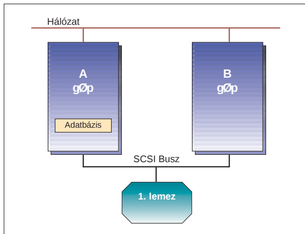
1. ábra Kétféles telep egy megosztott SCSI lemezzel
