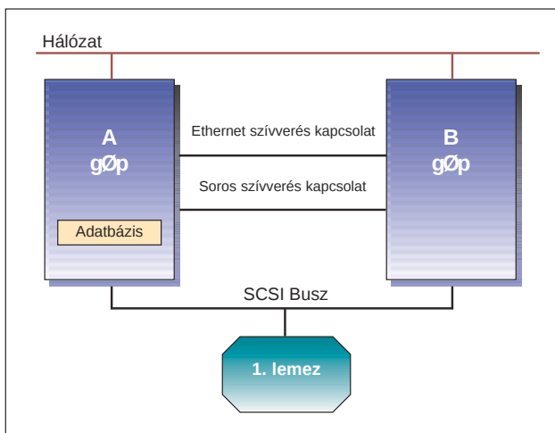
2. ábra Kétféles telep Ethernet és soros kapcsolattal
