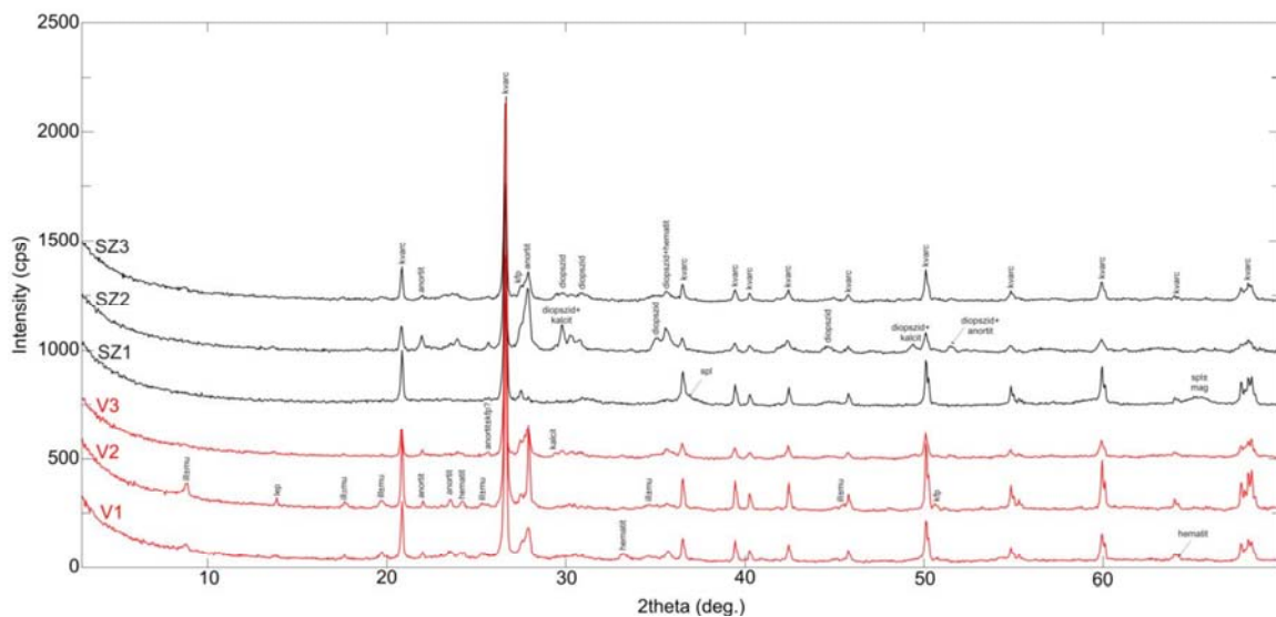
4. ábra: A kiválasztott reprezentatív minták XRD diffraktogramja (V1-3: vörös minták; SZ1: szemcsés helyi minta; SZ2-3: szürke minták)
