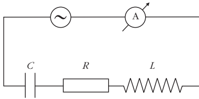
1. ábra. Egyszerű RLC-áramkör az L inuktivitás mérésére
