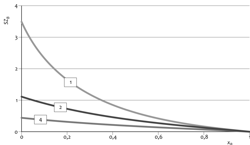
2. ábra • A szegregációs hányados függése a móltörttől, három dimenziómentes hőmérséklet-érték mellett, melyeket a görbéken tüntettünk fel ( T^* definíciójához lásd a Melléklet 6c egyenletét), a (8a–b) egyenletekkel számolva (paraméterek: \Omega^* = 0 és \Delta H_{COB}^{O*} = 10 )
