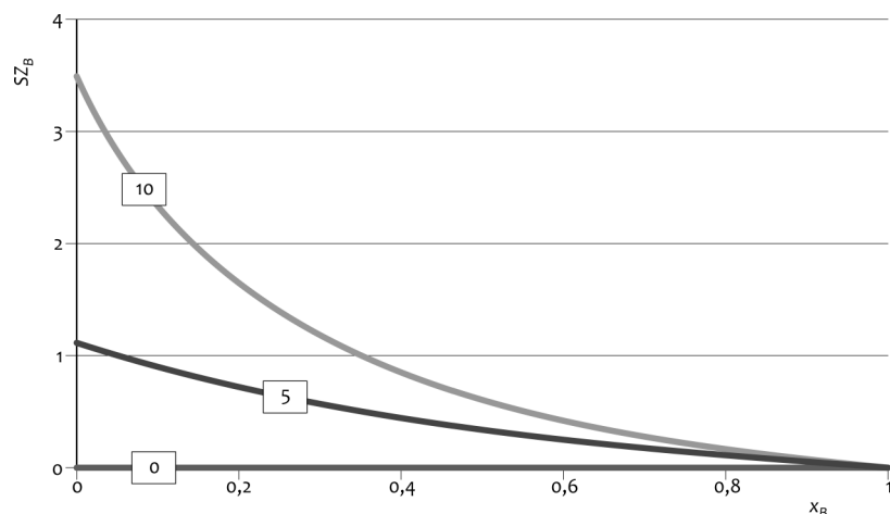
1. ábra • A szegregációs hányados függése a móltörttől, három \Delta H_{COB}^{O*} érték mellett (az értéket lásd a görbéken), a Melléklet (8a–b) egyenleteivel számolva (paraméterek: \Omega^* = 0 , T^* = 1 , az ábrán a \Delta H_{COB}^{O*} = 0 értékhez az SZ_B = 0 vízszintes vonal tartozik)
