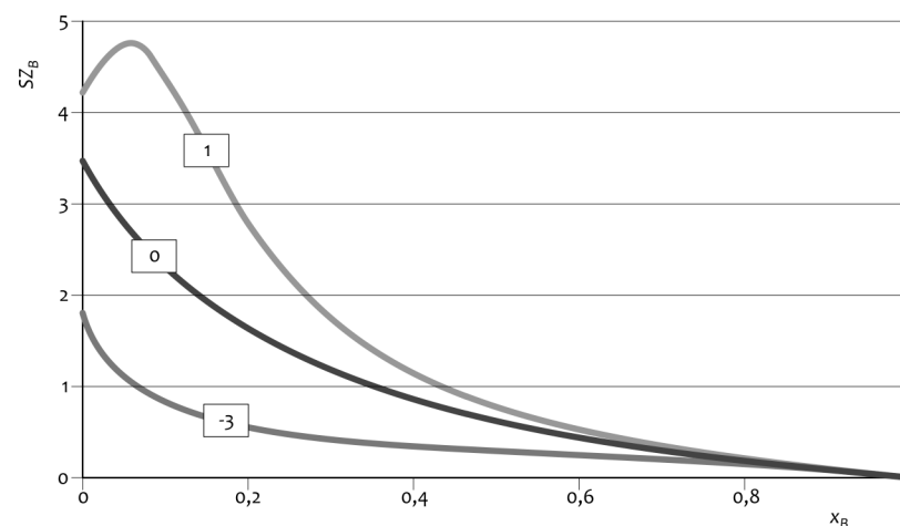
3. ábra • A szegregációs hányados függése a móltörttől, három kölcsönhatási energia ( \Omega^* ) érték mellett (az értéket lásd a görbéken), numerikusan számolva a Melléklet képleteiből (paraméterek: T^* = 1 , és \Delta H_{COB}^{O*} = 10 ).
