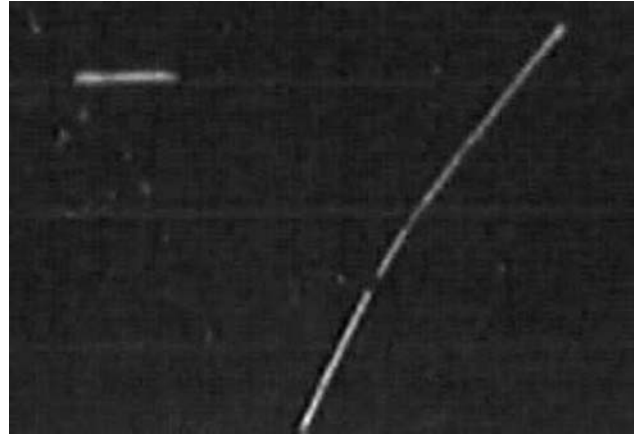
6. ábra. A ködkamrában megjelenő müon.
